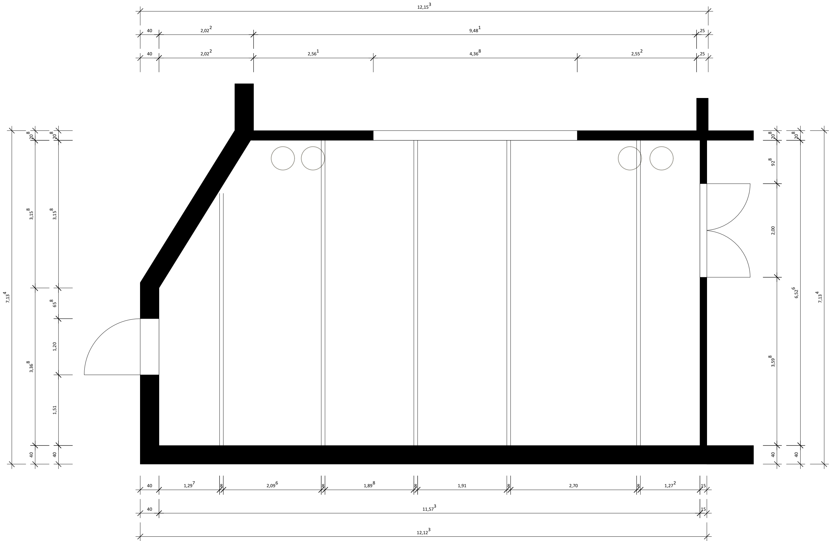
Draufsicht Raum mit Schwingboden M 1:50
